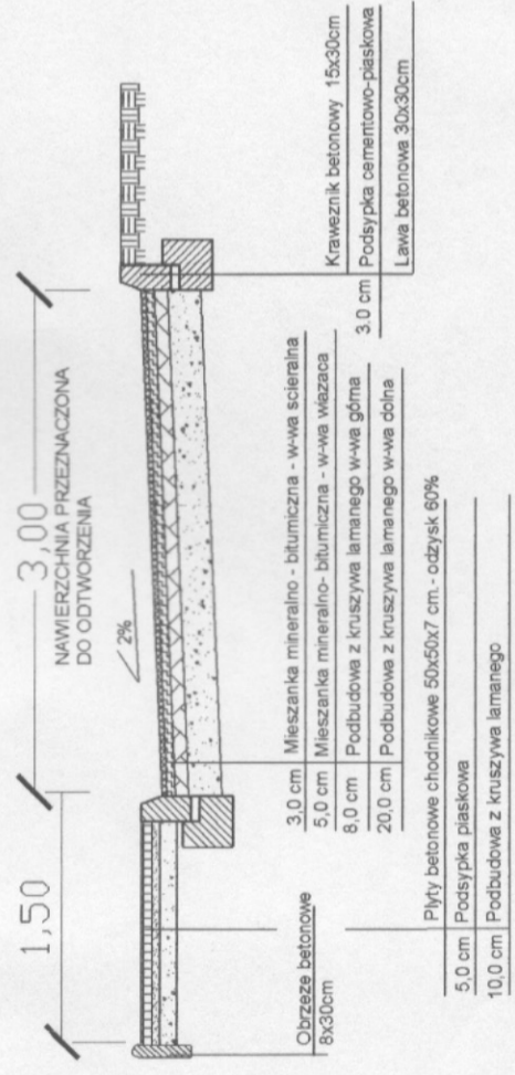
PRZEKROJ KONSTRUKCYJNY ULICY SPOKOJNEJ
